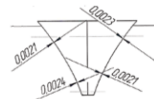
Протокол замера профиля долбяка и протяжки
