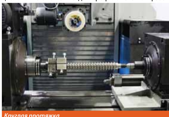
Круглая протяжка
