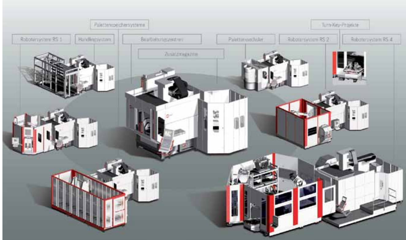
Рис. 5. Ассортимент систем автоматизации фирмы Hermle-Leibinger Systemtechnik GmbH
