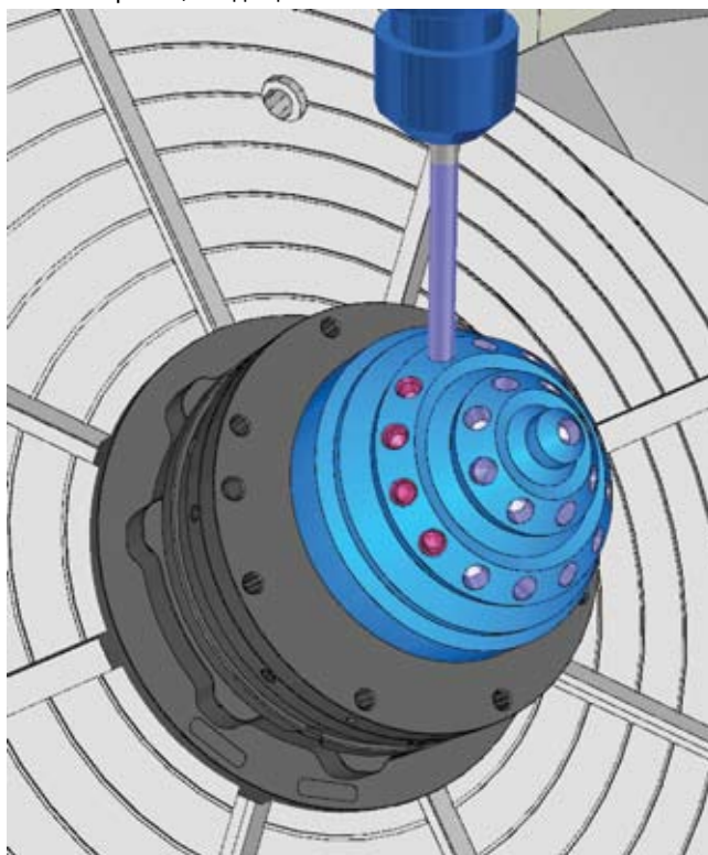
Рис. 3. В FeatureCAM 2015 поддерживается пятиосевая обработка массивов регулярно расположенных одинаковых отверстий
