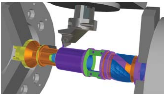
Рис. 1. Совершенствование разработки управляющих программ для сложных видов токарно-фрезерной обработки – одно из главных направлений развития CAM-системы FeatureCAM
