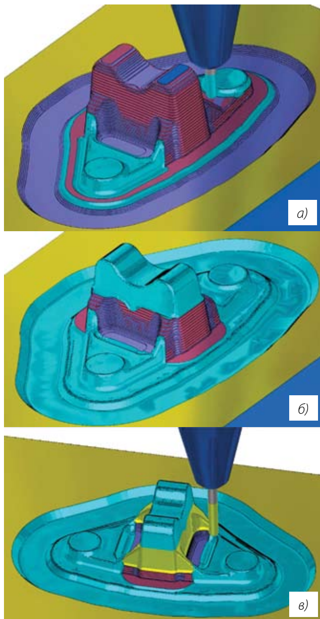
Рис. 5. 2015-я версия FeatureCAM позволяет с использованием трехосевых стратегий при помощи относительно короткого инструмента обработать максимально возможное количество материала (а, б), после чего снять остатки фрезой достаточной длины (в)
