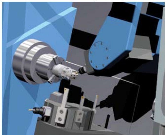
Рис. 2. CAM-система FeatureCAM позволяет программировать комбинированные виды обработки приводным инструментом (B-осью)
