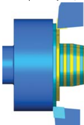
Рис. 6. Токарный модуль FeatureCAM 2015 позволяет программировать обработку поверхности одновременно двумя резцами (если станок оснащен нижней револьверной головкой)
