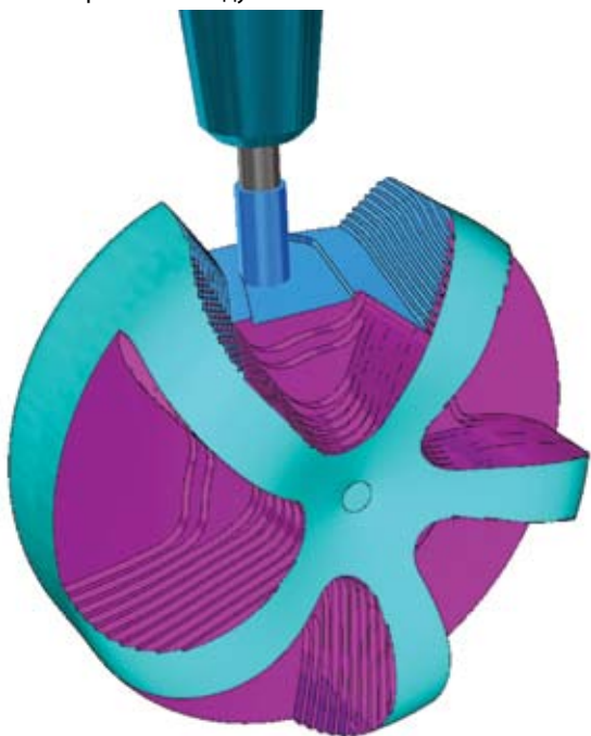
Рис. 4. FeatureCAM 2015 позволяет после каждой операции сохранять текущую 3D-модель остатка материала для ее последующего использования в качестве заготовки
