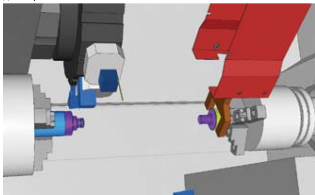
Рис. 7. В FeatureCAM 2015 реализована поддержка программируемых деталями-уловителей и захватного устройства для противощпинделя
