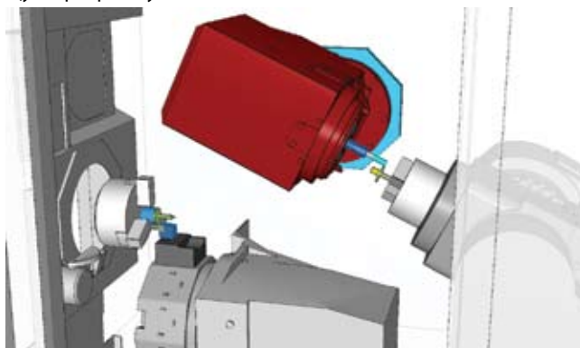
Рис. 8. FeatureCAM 2015 поддерживает 3D-симуляцию и постпроцессирование управляющих программ для станков сложной компоновки, в том числе, Mori Seiki NTX1000 оснащенного поворотным противощпинделем
