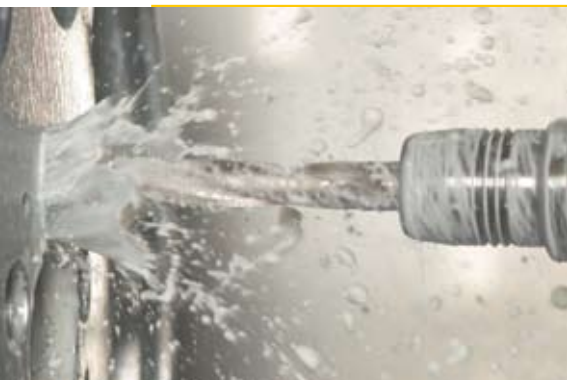
Рис. 6. Сверление алюминиевой заготовки
