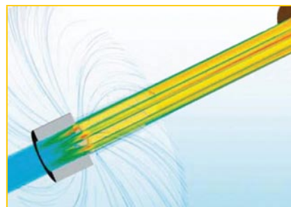
Рис. 3. Без потерь по лезвию: Несмотря на высокую частоту вращения и связанную с ней экстремальную центробежную силу, СОЖ протекает почти без потерь по шейке инструмента до режущей кромки в отверстие. Только при попадании на заготовку происходят минимальные боковые потери
